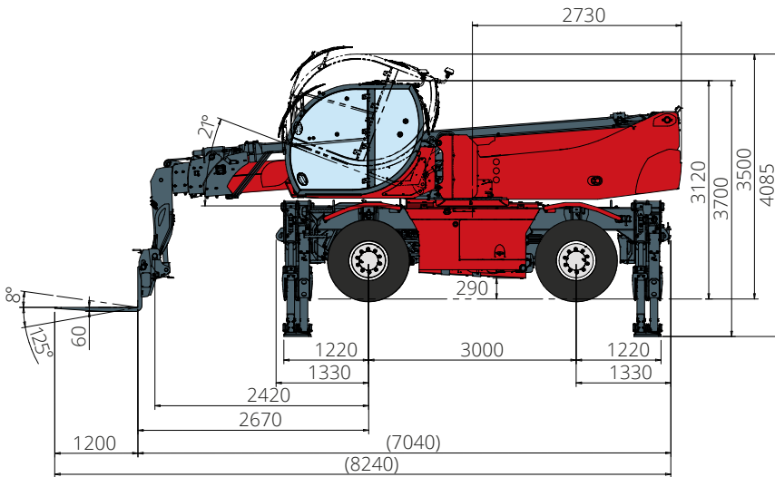
SEITENANSICHT
