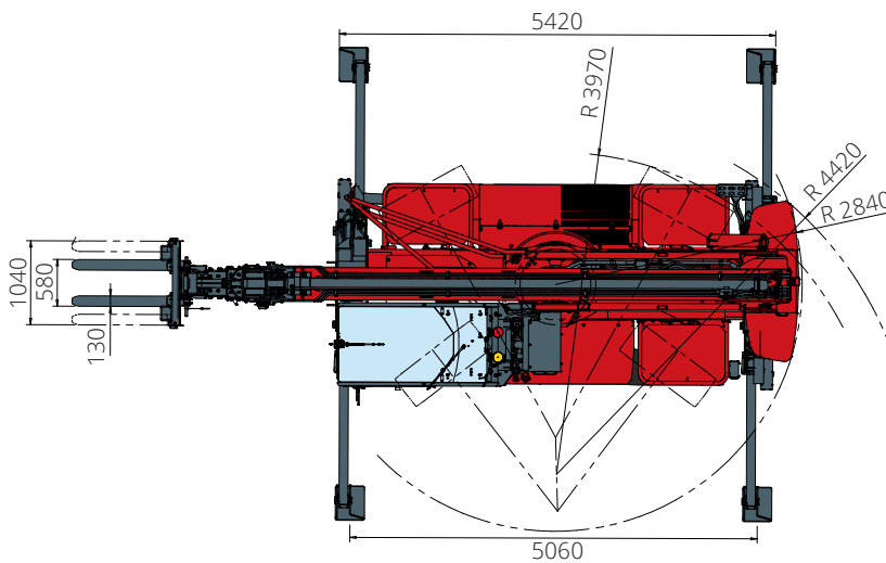
AUFSICHT
