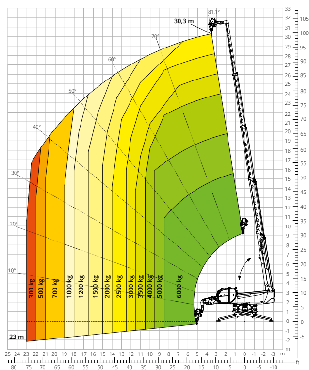
Diagramma portate con ARGANO 6.000 kg ATT - 02 - 004
