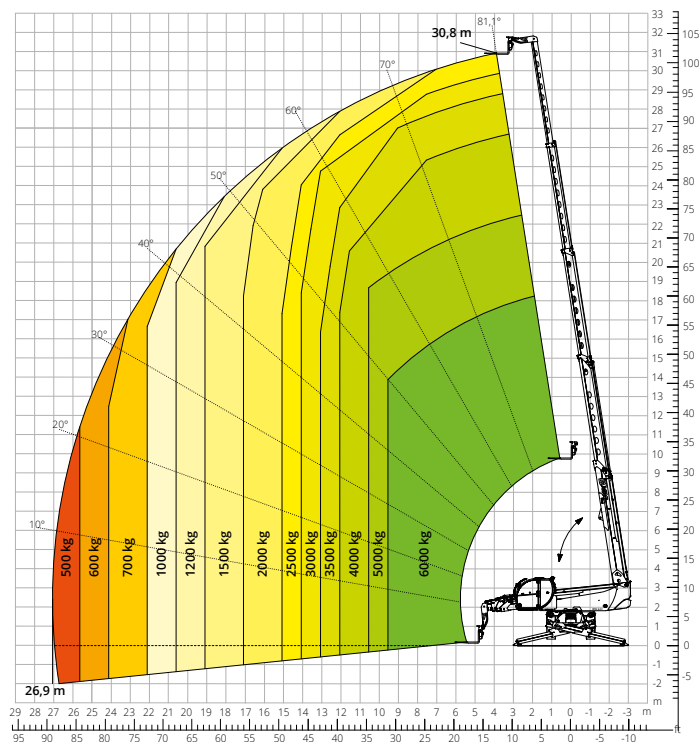
Diagramma portate con STABILIZZATORI ESTESI 360° ATT-03-004
