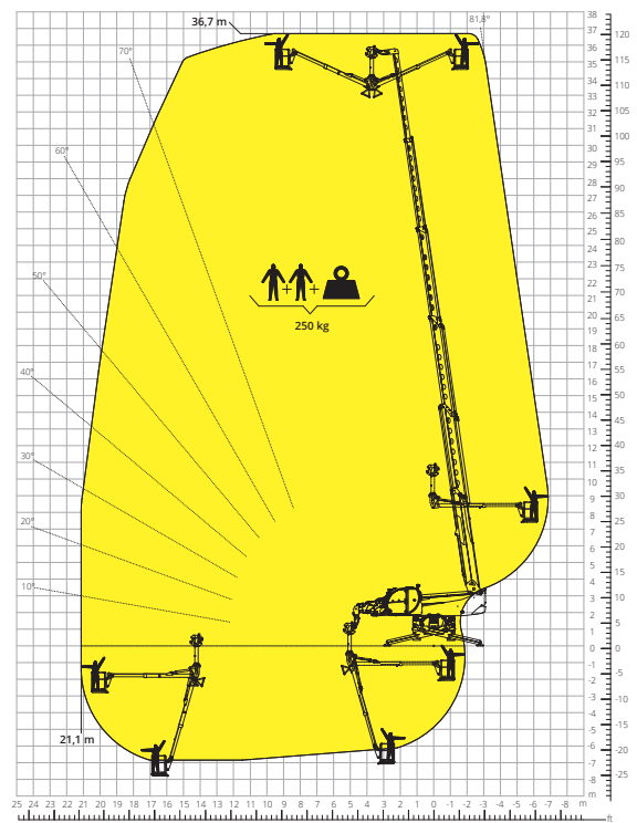
Diagram obciążeń z PLATFORMĄ MOSTOWĄ - NEGATYW ATT - 01 - 024
