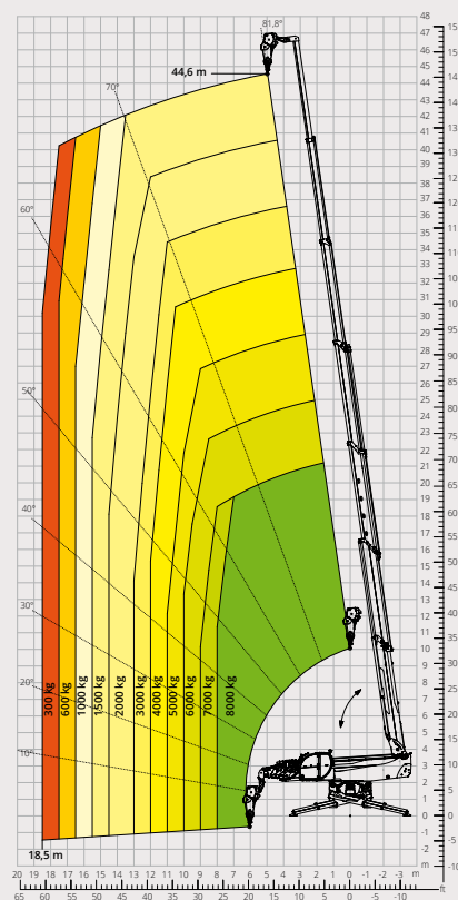
Lastdiagramm mit SEILWINDE 8.000 kg - M2 ATT - 02 - 006
