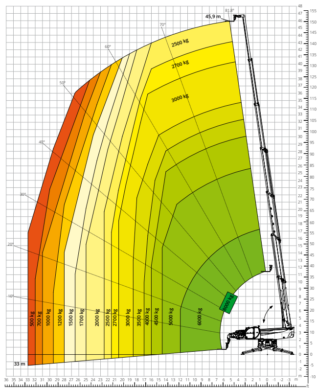
Lastdiagramm mit AUSGEFAHRENEN STÜTZEN 360° - M1 ATT - 03 - 007
