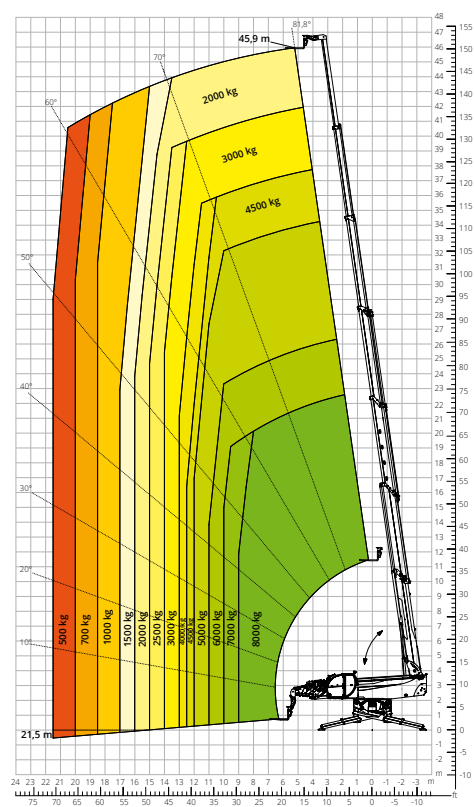
Lastdiagramm mit AUSGEFAHRENEN STÜTZEN 360° - M2 ATT - 03 - 007
