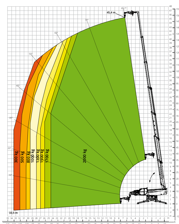
Lastdiagramm mit AUSLEGER MIT SEILWINDE 2.000 kg ATT - 04 - 015
