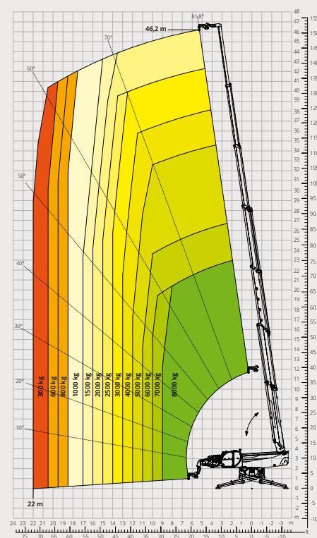
Lastdiagramm mit LASTHAKEN 8.000 kg - M2 ATT - 05 - 003
