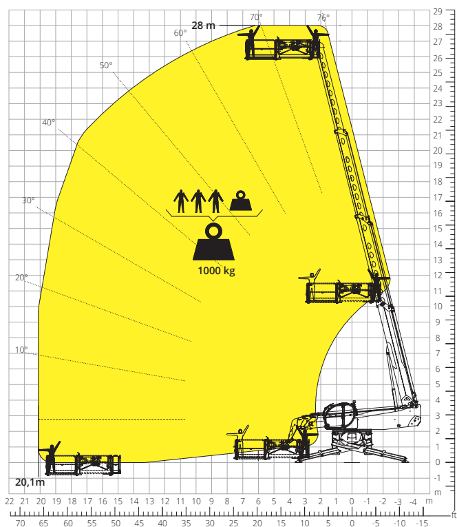
Diagram obciążeń z PLATFORMĄ ROZSUWANĄ DO DACHÓW, 1.000 kg ATT - 01 - 020
