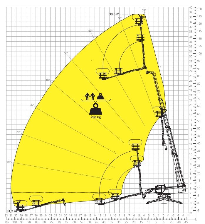
Diagram obciążeń z PLATFORMĄ TELESKOPOWĄ, 200 kg - 10 m ATT - 01 - 022
