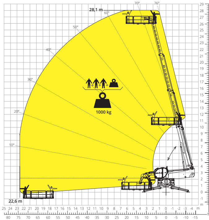
Diagram obciążeń z PLATFORMĄ ROZSUWANĄ DO DACHÓW, 1.000 kg ATT - 01 - 020
