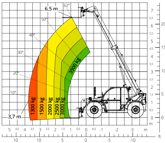
Diagrama de carga en estabilizadores extendidos
