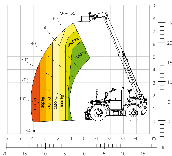
Lastdiagramm frontal auf Reifen
