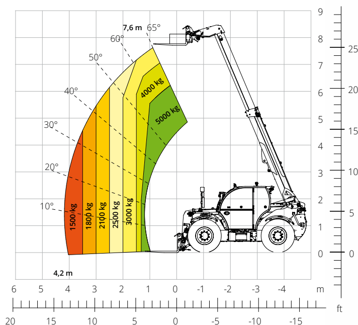
Diagrama de carga en estabilizadores extendidos
