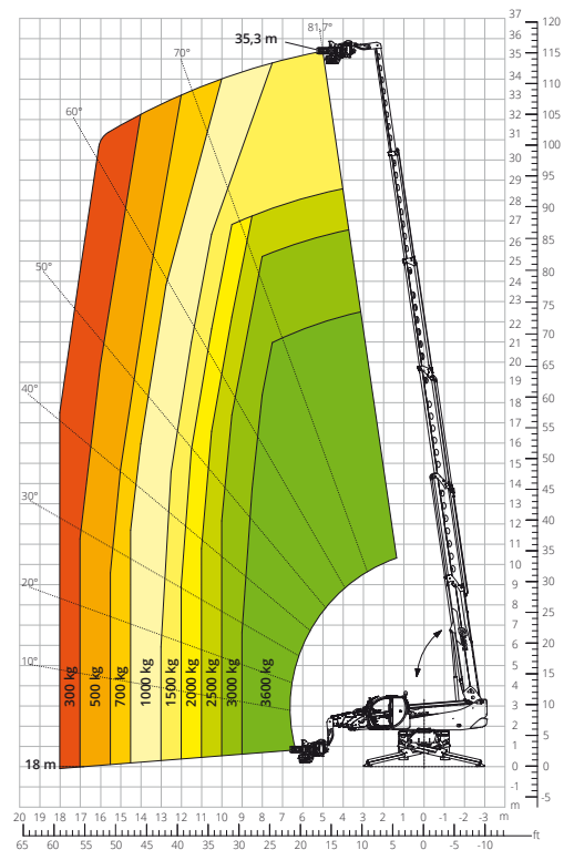
Lastdiagramm mit FÄLLKOPF ATT - 08 - 001
